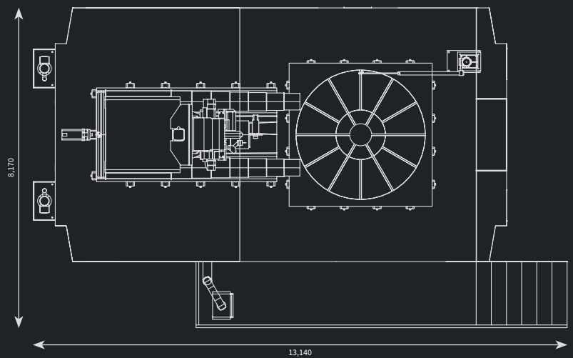
RAPID 6000: 俯视图
